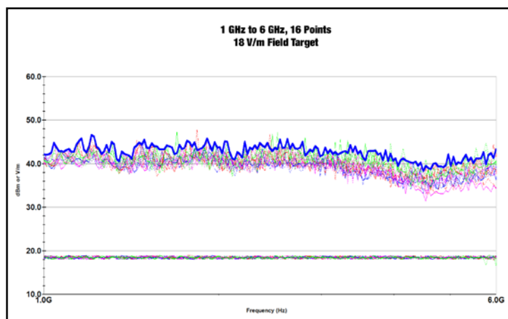
18V/m CWをターゲット・フィールドにした実測電力(水平偏波)
